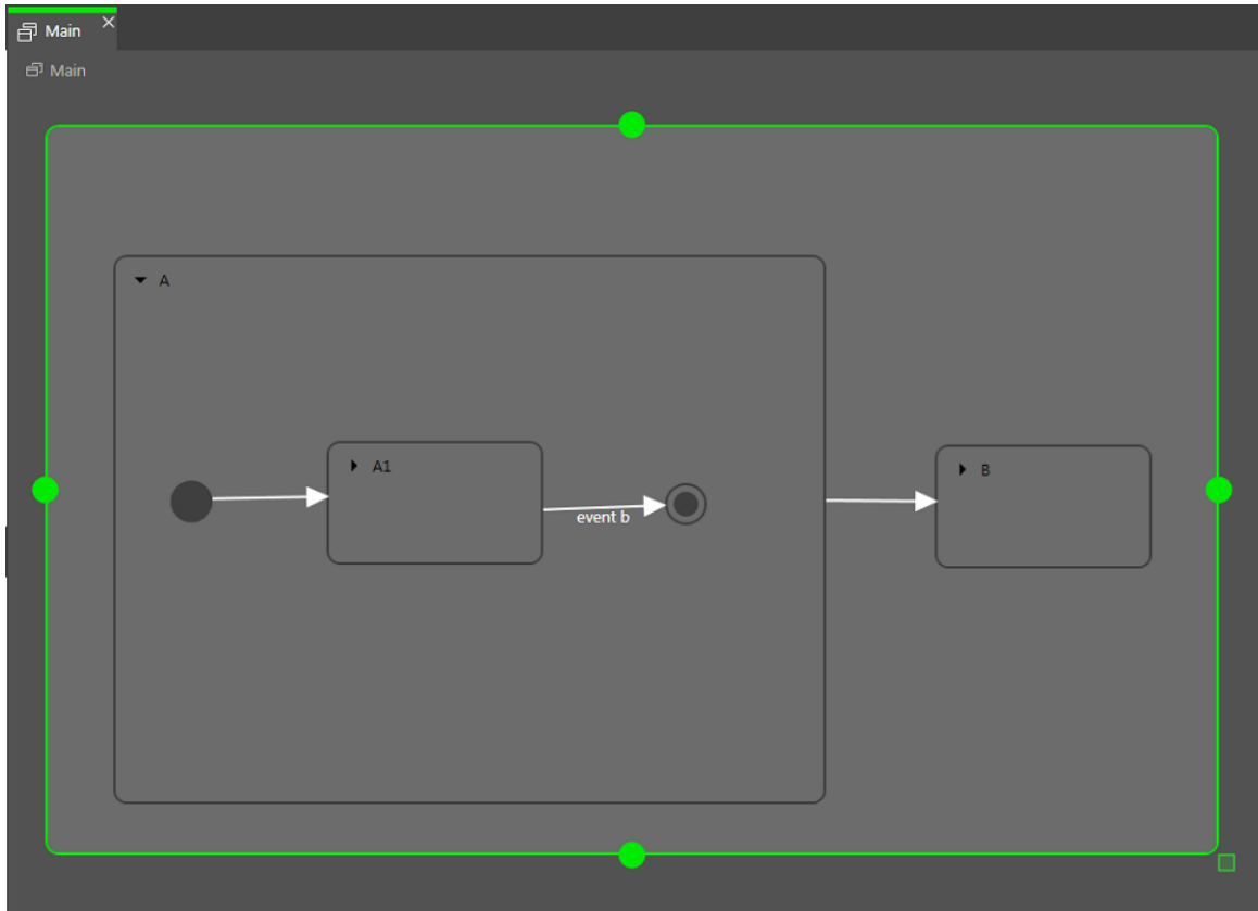
그림 6.23. 복합 상태 내의 최종 상태 사용법
