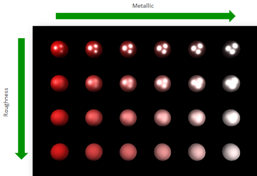
그림 15.1. 물리적 기반 재료의 예
