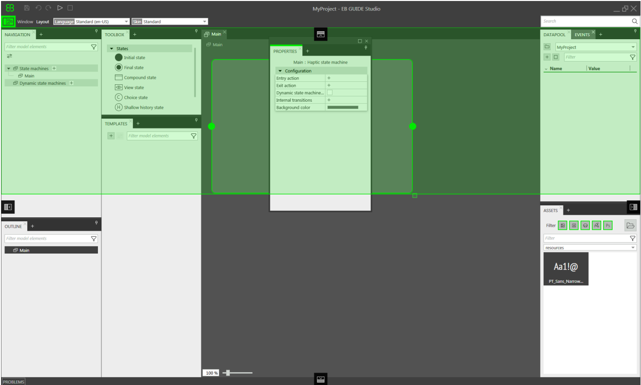
그림 6.11. 도킹 제어 및 실시간 미리 보기
