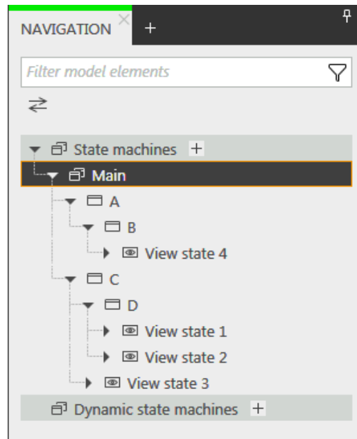
그림 6.21. 트리로 표시되는 상태 계층
