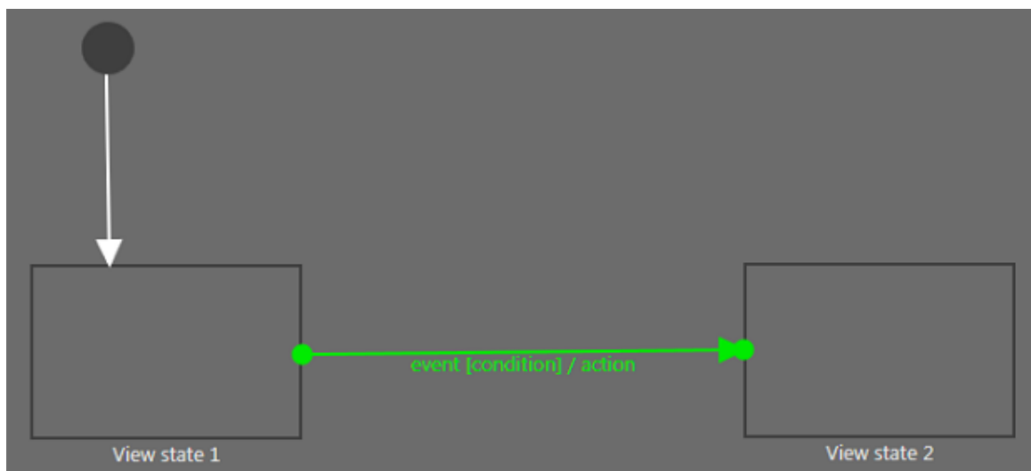
그림 6.27. 전이
