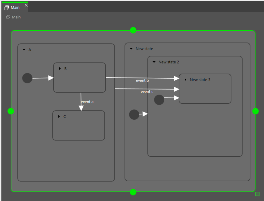
그림 6.30. 전이 실행
