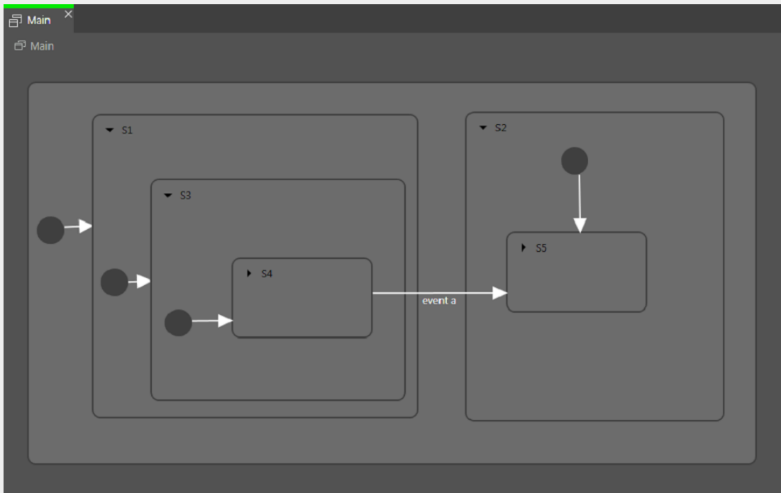
그림 6.31. 전이 실행
