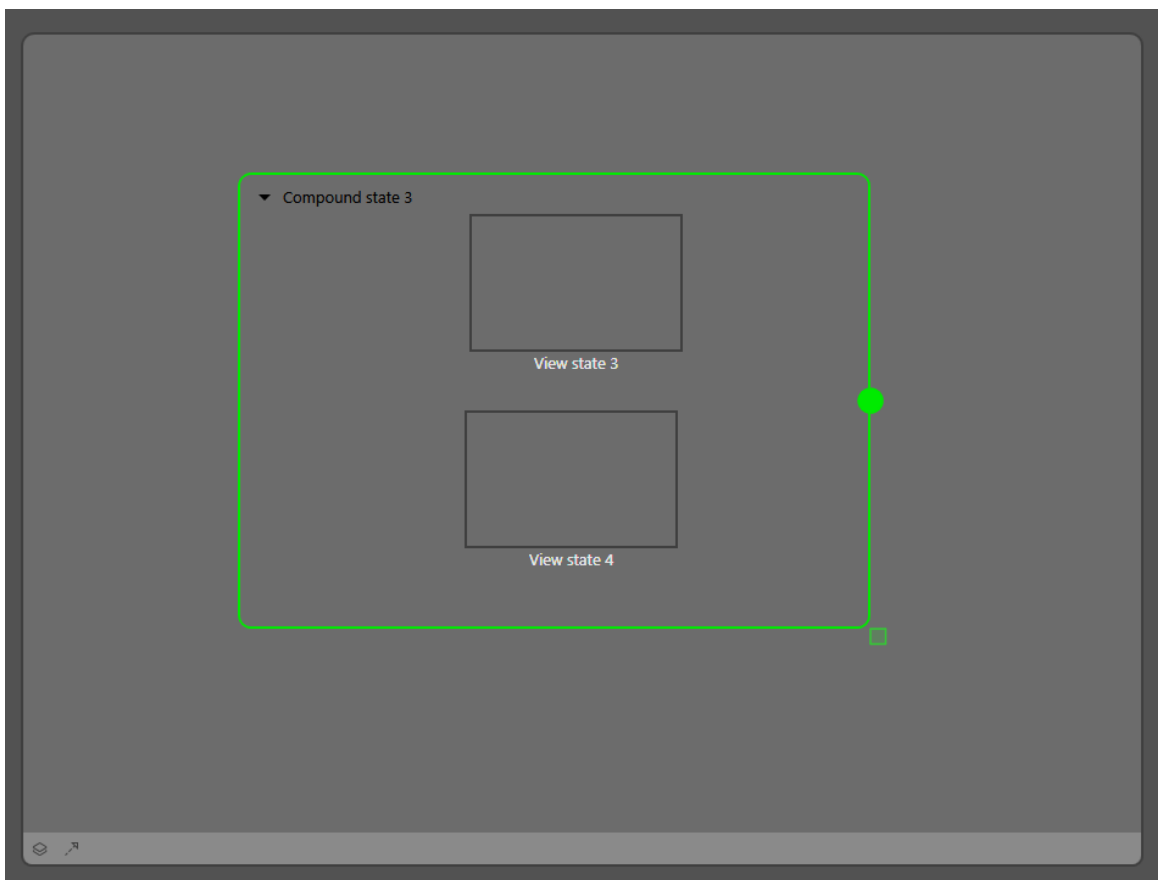
그림 6.20. 복합 상태
