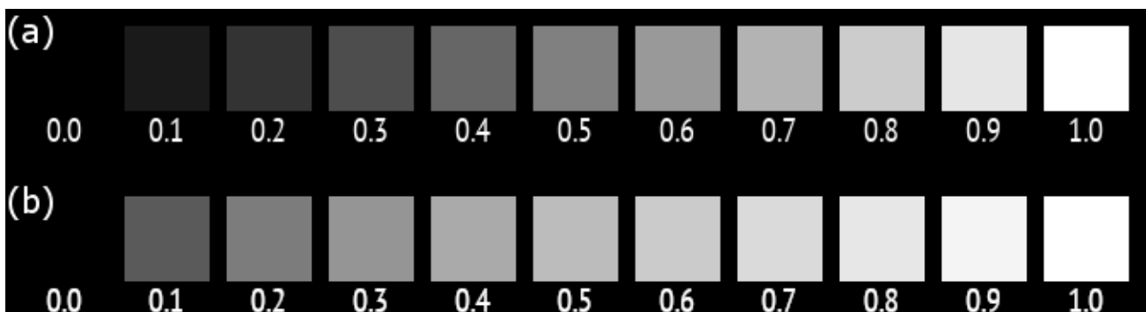
그림 6.13. 감마의 예
