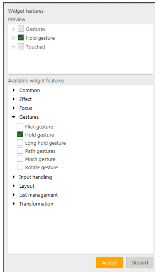
그림 6.35. 위젯 피쳐
