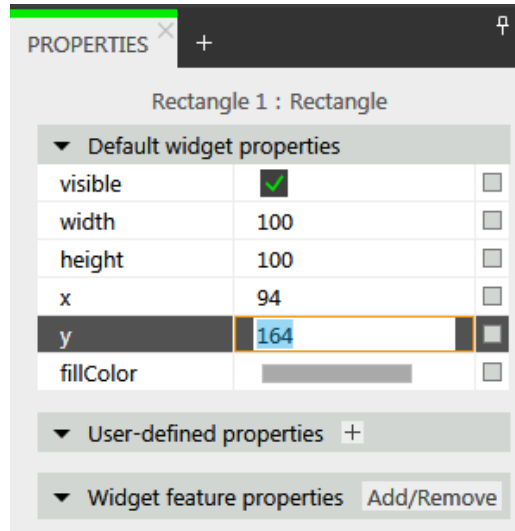
그림 8.3. 사각형의 속성
