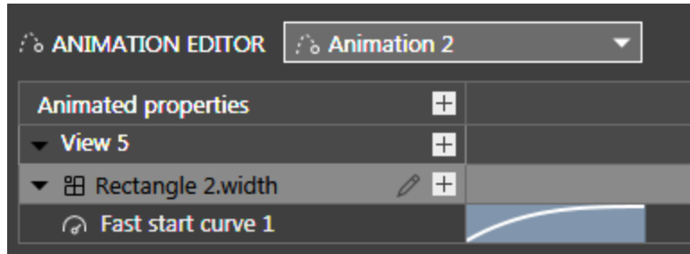
그림 6.8. 애니메이션 편집기
