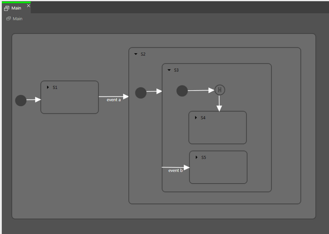
그림 6.32. 전이 실행
