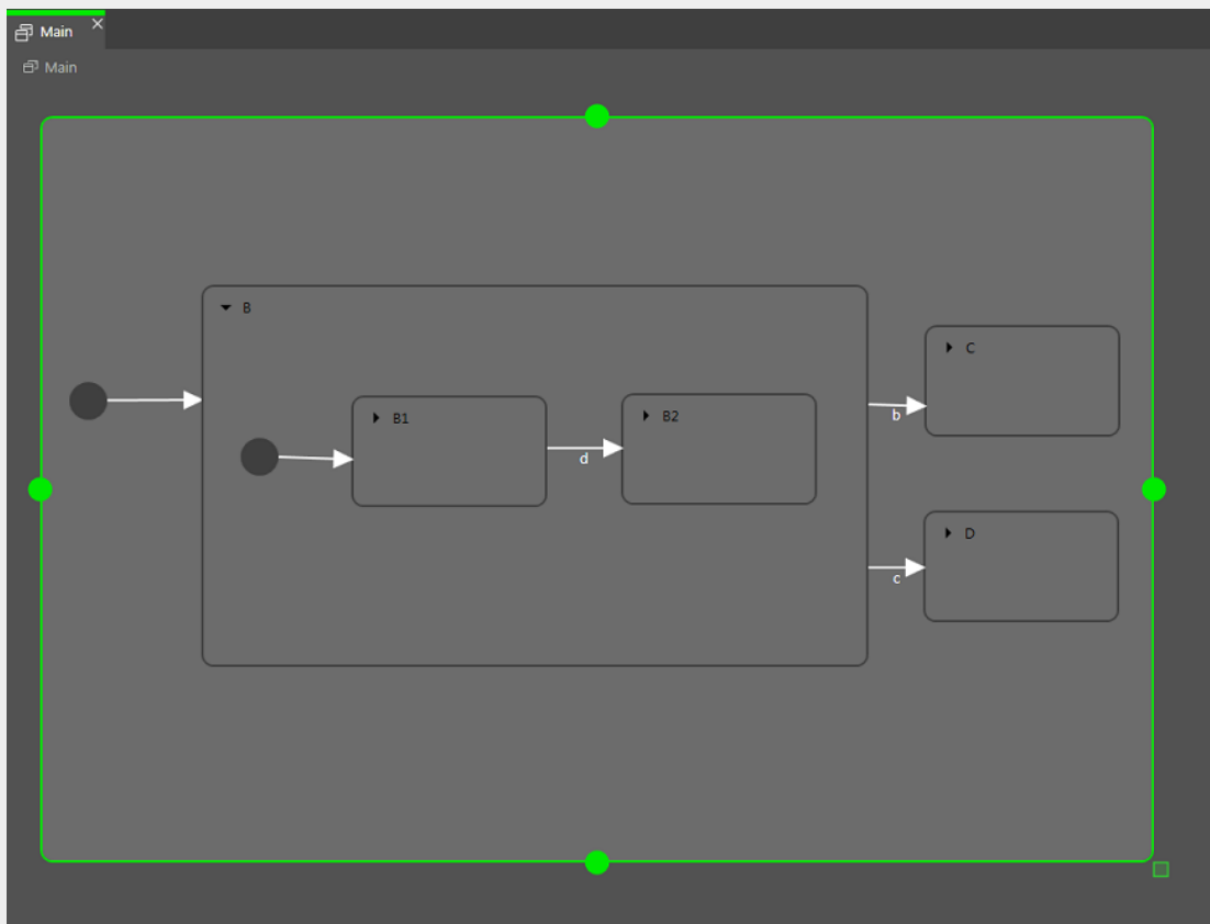
그림 6.28. 전이 상속
