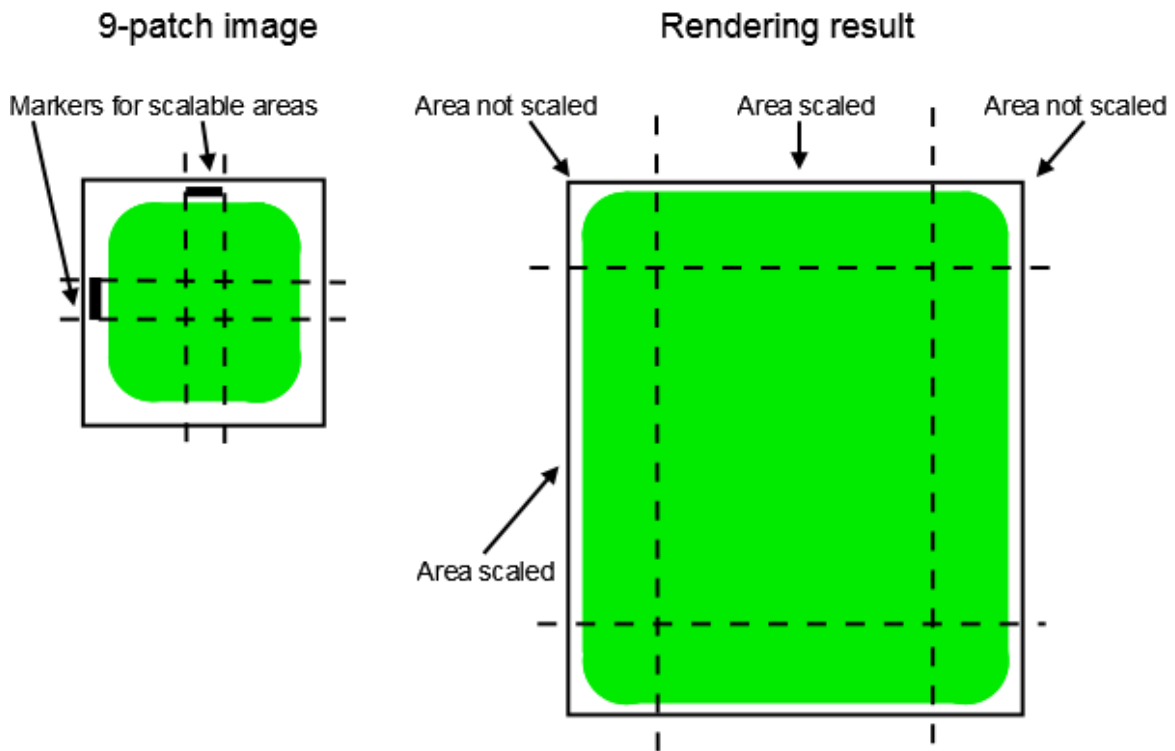
그림 6.18. 나인패치 예제
