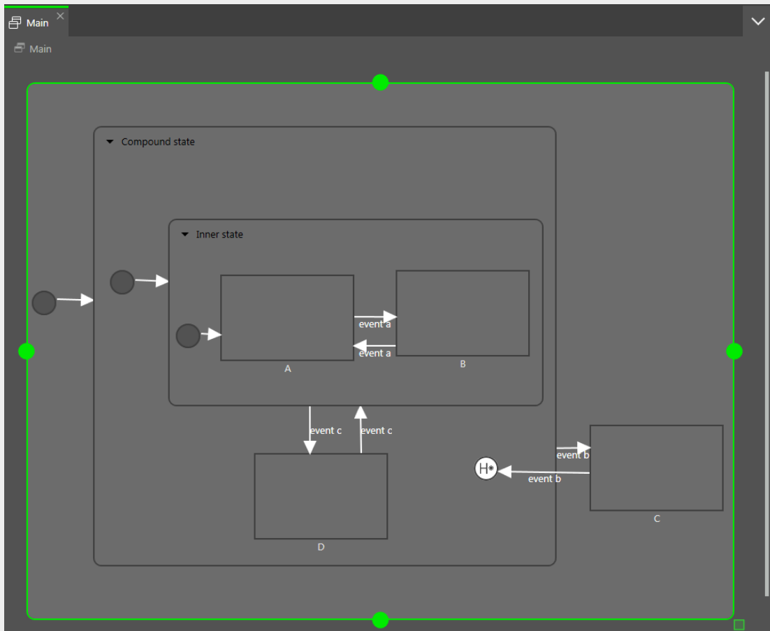
그림 6.26. 깊은 이력 상태
