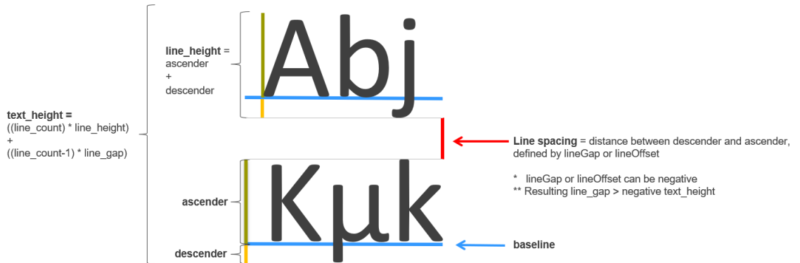
그림 8.7. 텍스트 높이, 줄 높이 및 줄 간격 계산
