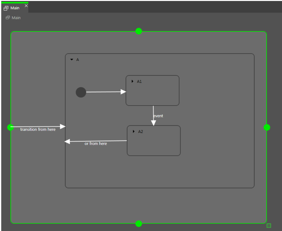
그림 6.22. 초기 상태의 예
