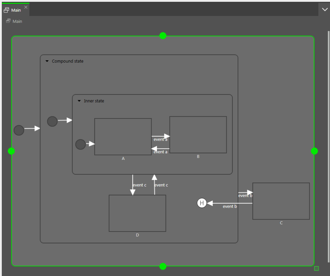
그림 6.25. 얇은 이력 상태
