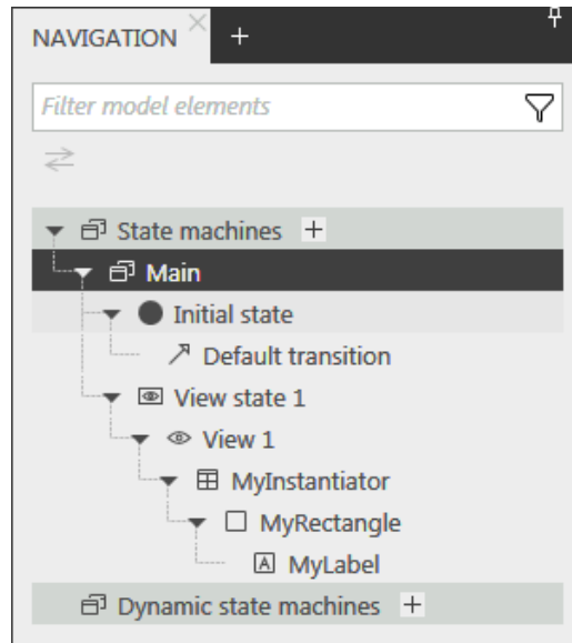
그림 14.5. 인스턴스화기가 포함된 위젯 계층
