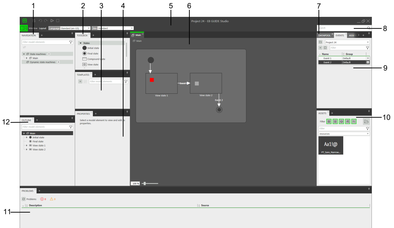
그림 6.3. 영역 및 구성 요소가 포함된 프로젝트 편집자
