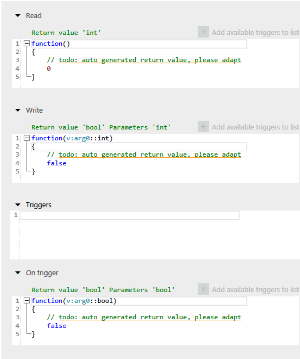
그림 6.19. EB GUIDE Studio의 EB GUIDE 스크립트 편집기
