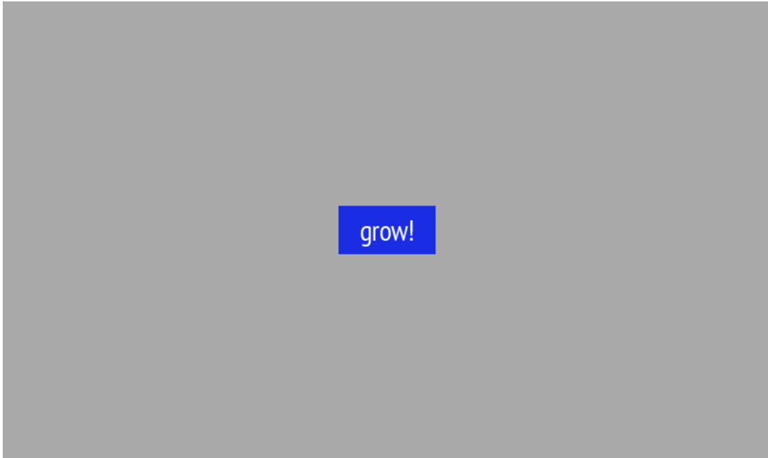
그림 14.4. 결과
