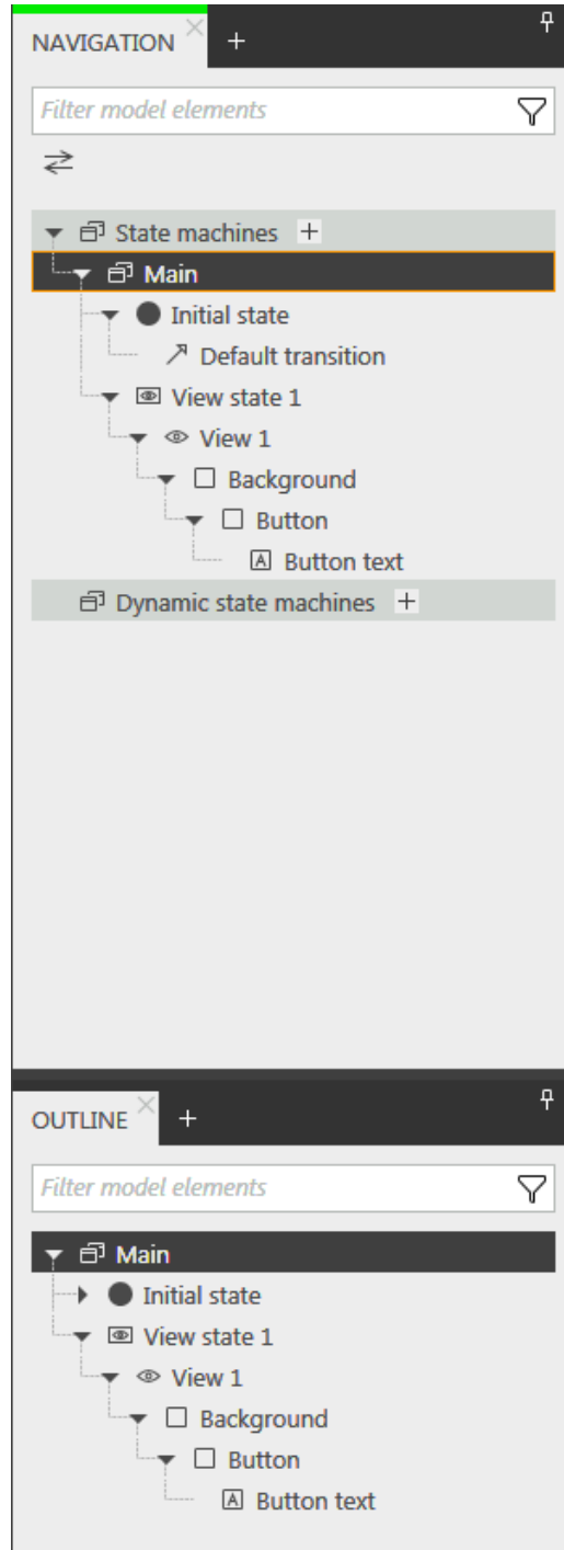
그림 14.3. 위젯 계층
