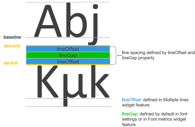
그림 8.8. 다음에 의해 정의된 줄 간격: lineOffset 및 lineGap
