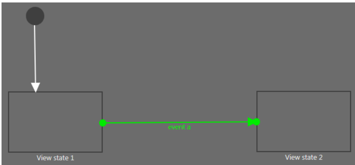
그림 7.4. 트리거가 포함된 전이
