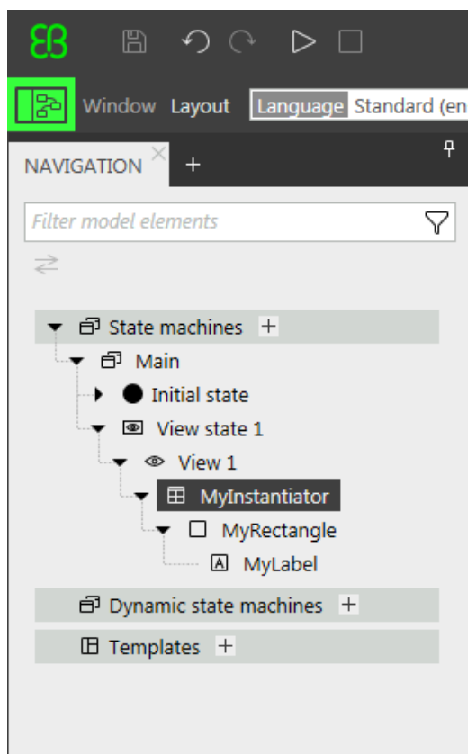
図11.5 インスタシエータを含むウィジェット階層
