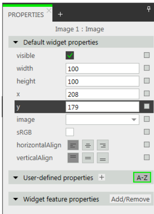
図6.6 ウィジェットのプロパティが表示された[プロパティ]コンポーネント
