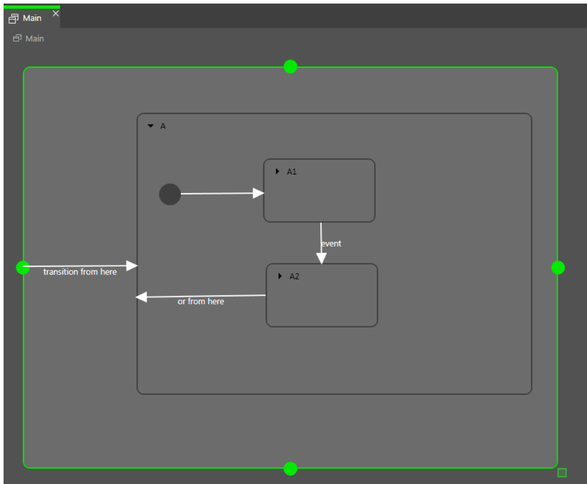
図6.18 初期状態の例
