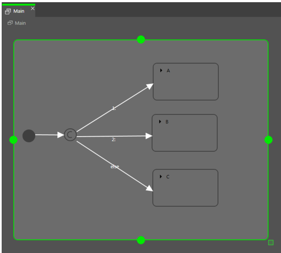
図6.20 入力遷移と出力遷移を持つ選択状態
