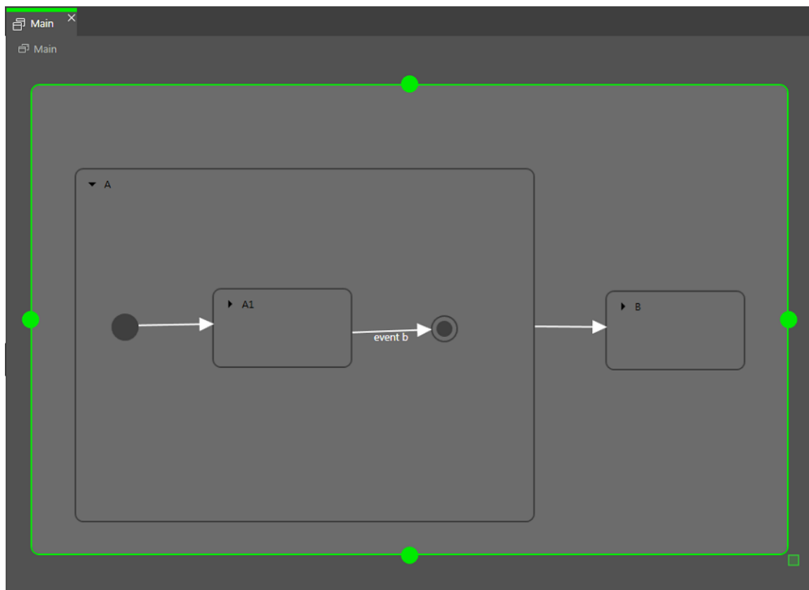
図6.19 混合状態内での最終状態の使用方法
