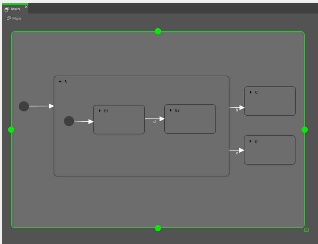
図6.25 遷移のオーバーライド
