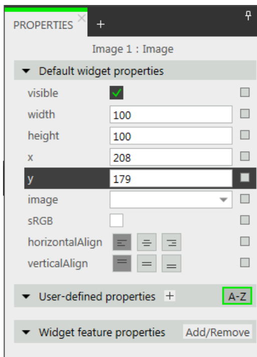
図8.3 イメージのプロパティ
