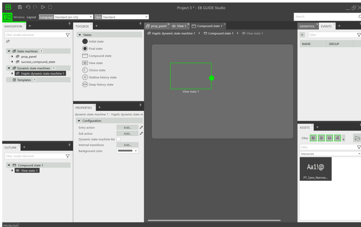
図7.1 入れ子のビューステートを持つ混合ステート
