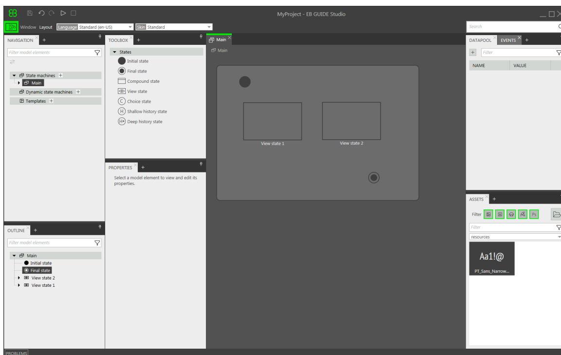
Figure 5.3. ステートが表示されたプロジェクトエディター
