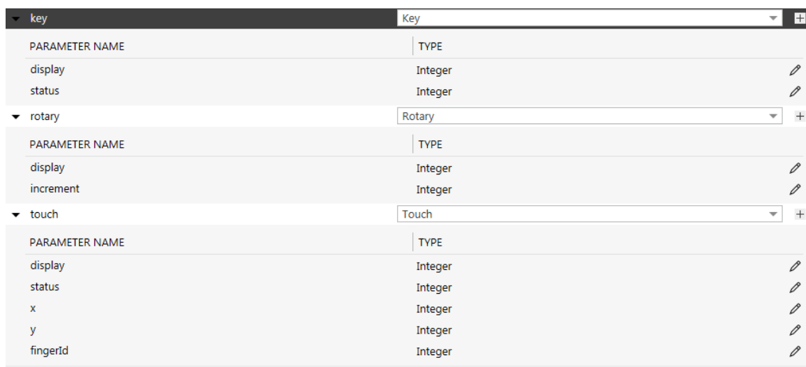
図6.11 イベントグループおよびイベントIDの例
