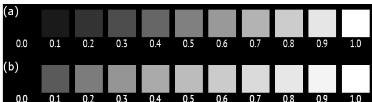
図6.12 ガンマの例
