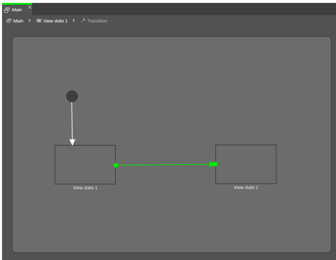
図7.3 遷移
