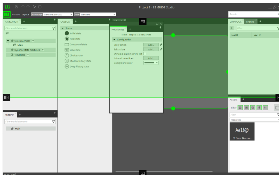
図6.9 ドッキングコントロールとライブプレビュー
