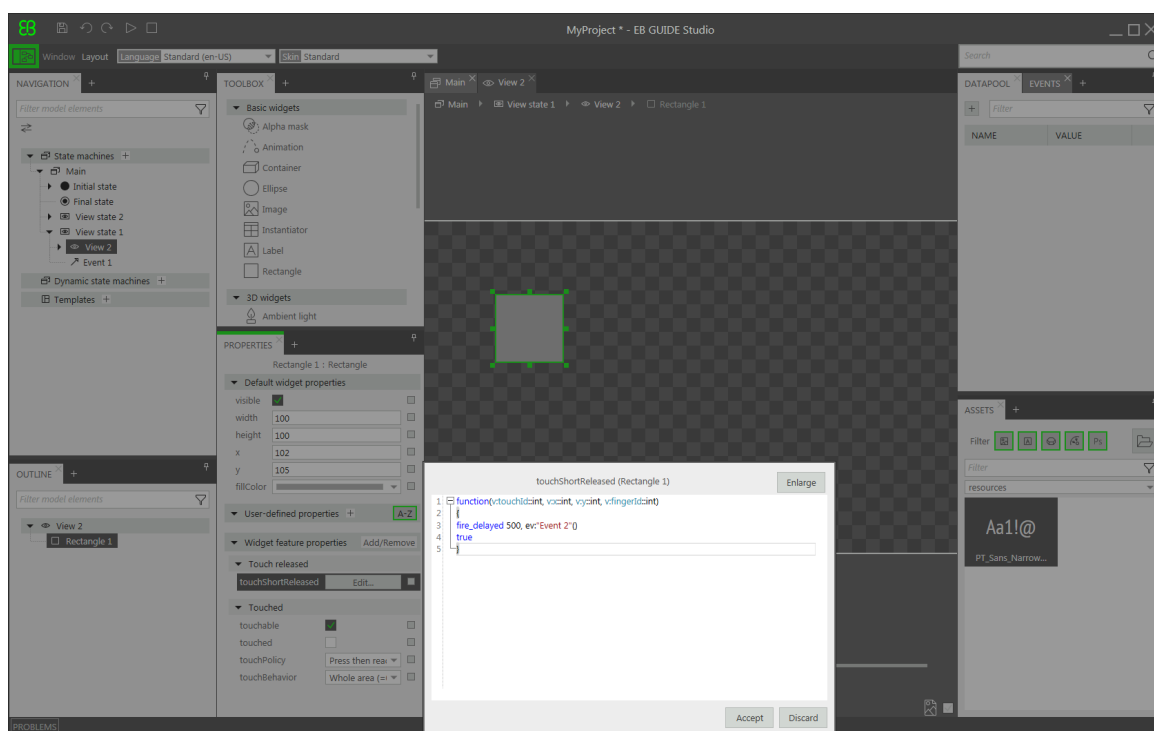
Figure 5.5. EB GUIDEスクリプトを持つウィジェットプロパティ
