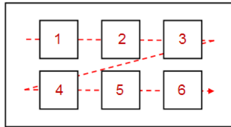
図6.32 [自動フォーカス]ウィジェット機能のポリシー
