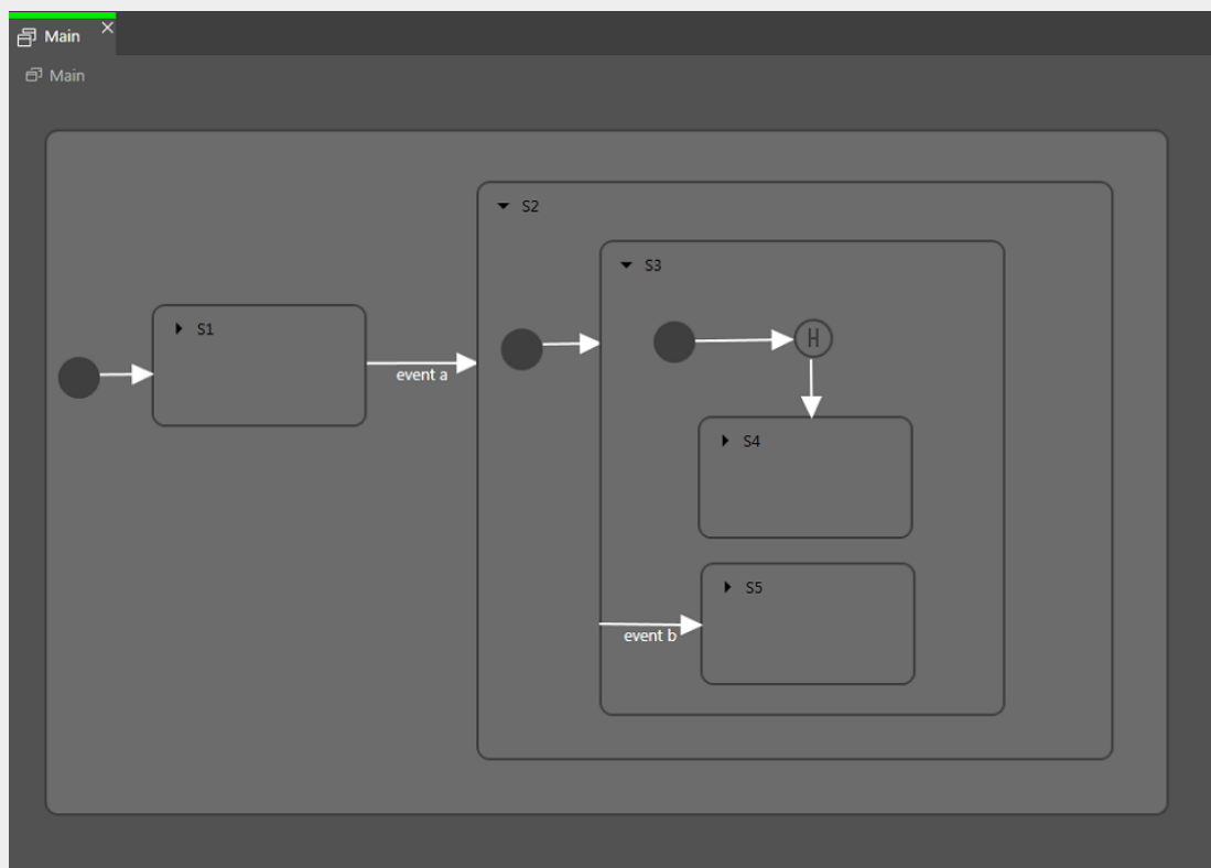
図6.28 遷移の実行
