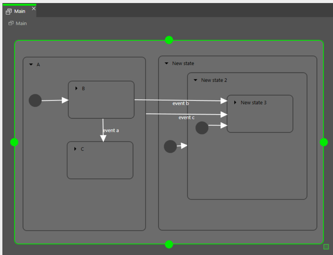
図6.26 遷移の実行
