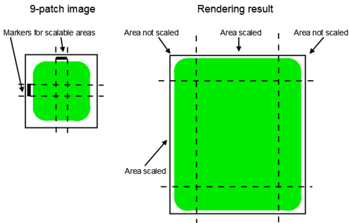
図6.14 9-patchの例
