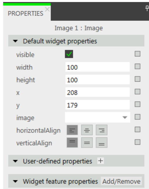
图 8.2. 图像的属性
