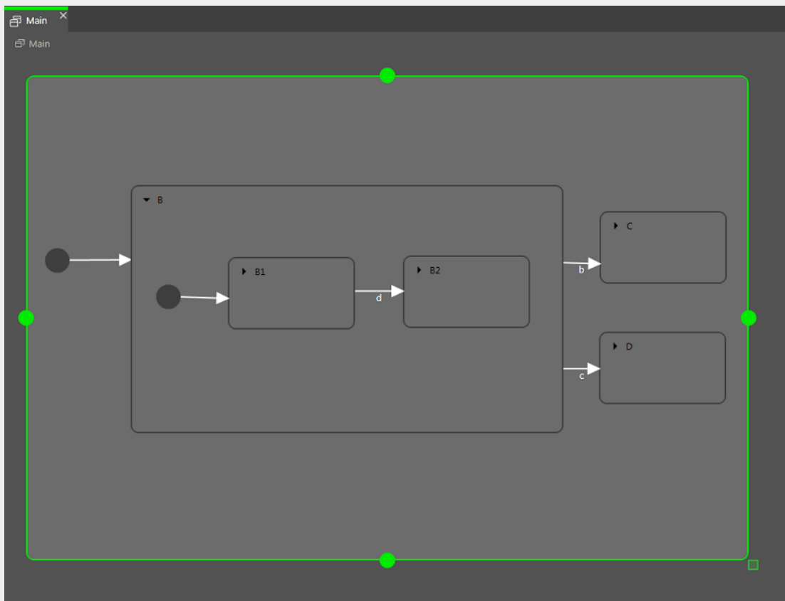
图 6.20. 转换继承
