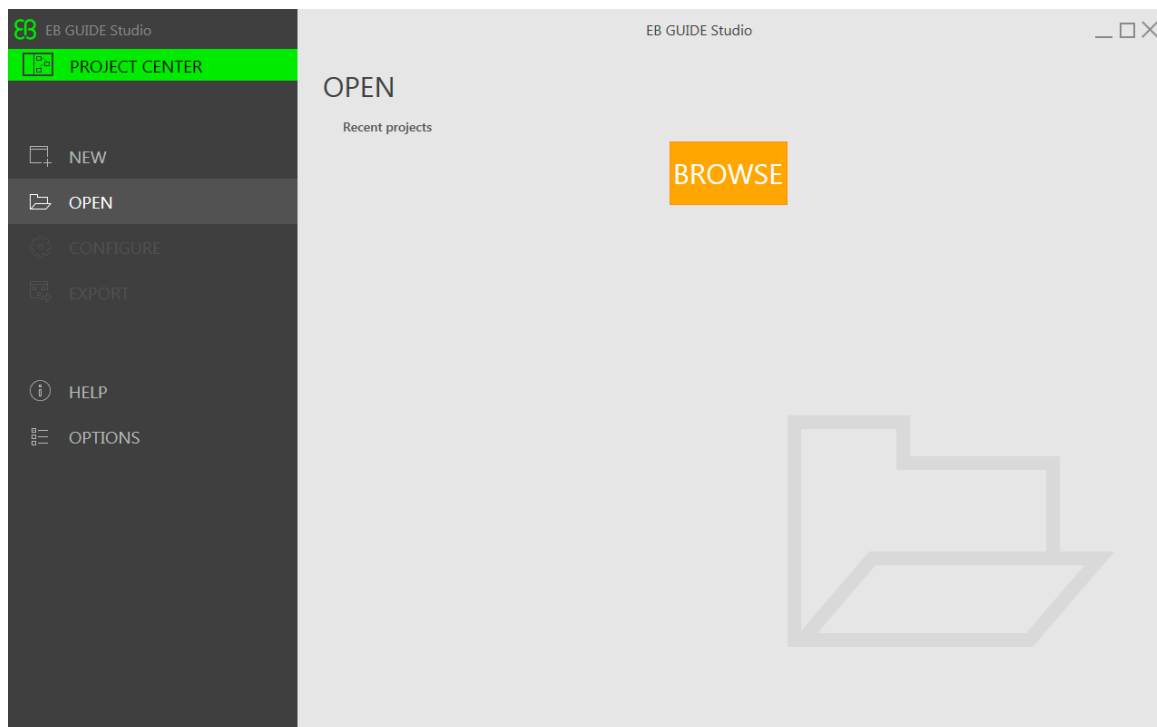
图 5.1. 项目中心
