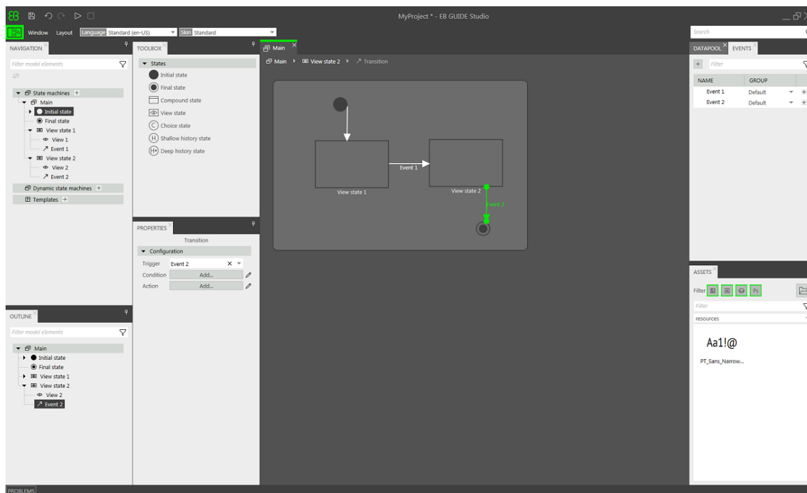
図5.4 イベントを伴う遷移でリンクされた状態
