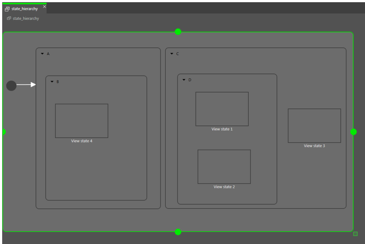
図6.12 混合状態
