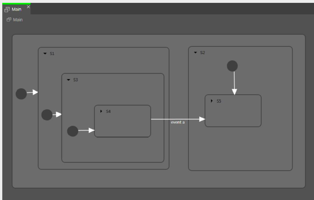
図6.23 遷移の実行
