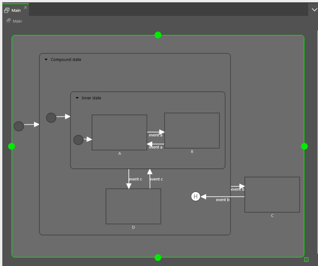
図6.17 浅い履歴状態
