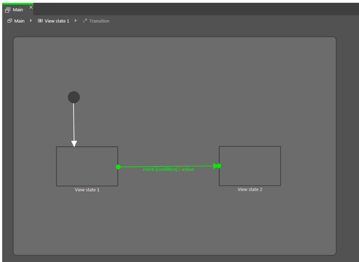
図6.19 遷移
